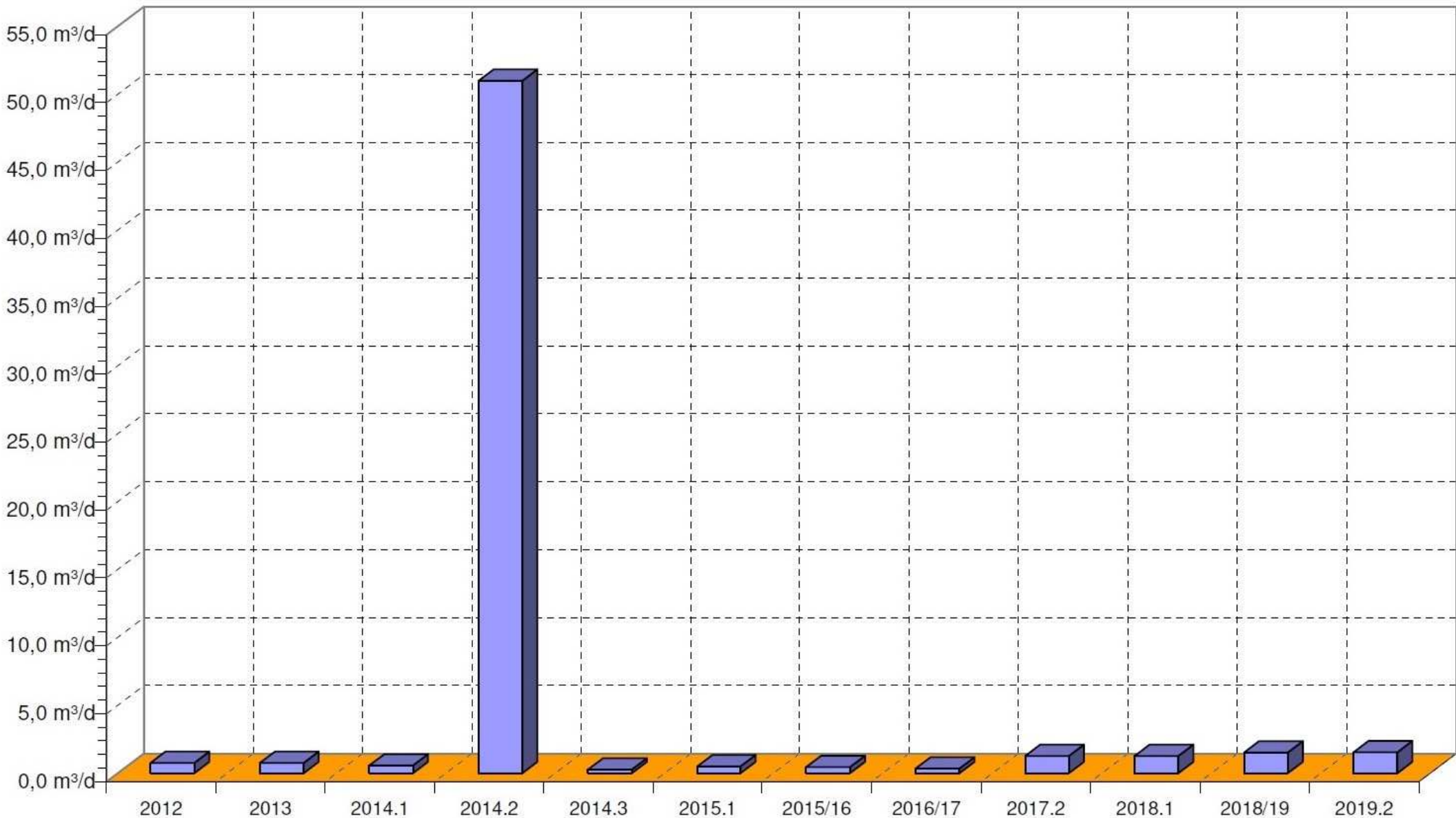
Bild 17: Darstellung der durchschnittlichen täglichen Trinkwasser-Verbrauchswerte für Ablesezyklen. Zu erkennen ist der Mehrverbrauch durch die Inbetriebnahme des Fitnessstudios ab 2016
